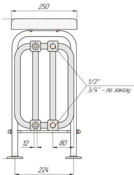
"Завалинка РС 4", боковое подключение монтажная схема. Присоединительная резьба - 1/2" (3/4" - по заказу)
