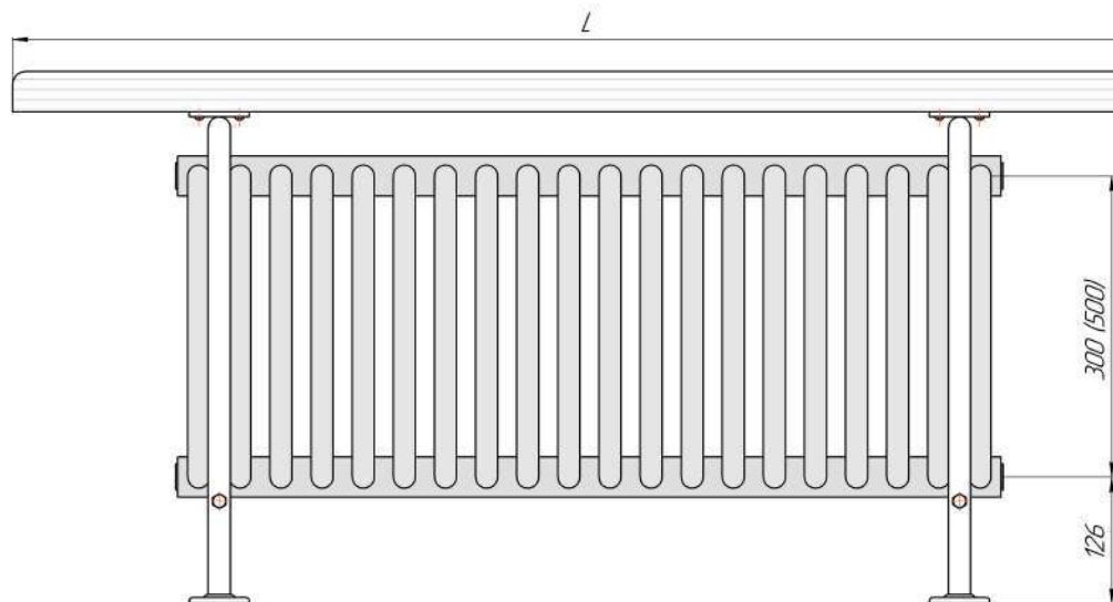
"Завалинка РС 4", боковое подключение монтажная схема. Присоединительная резьба - 1/2" (3/4" - по заказу)
