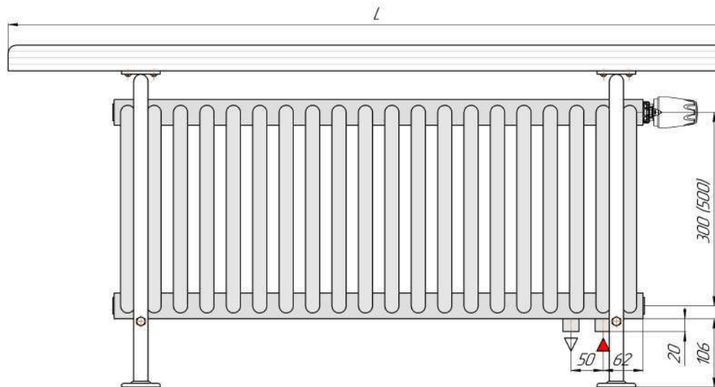
"Завалинка РС 4 нп", нижнее подключение, монтажная схема. Присоединительная резьба - внутренняя 1/2"
